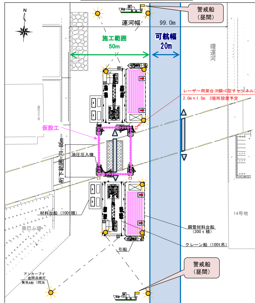
平面図 (仮設工)
